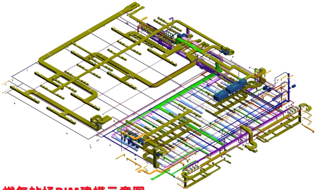
燃气站场BIM建模示意图
